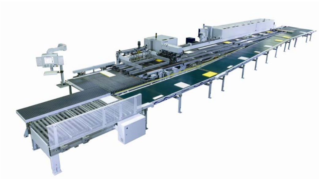
Bild 2: Anlage zur Fertigung von Möbelteilen in Losgröße 1
