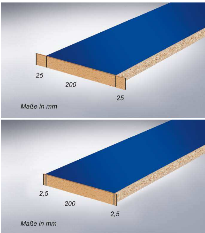
Bild 2: Erhebliche Reduzierung des Kantenabfalls mit der Servokantenzuführung: Die Kanten werden mit geringstem Überstand zur Werkstückecke an der Vorder- und Hinterkante zugeführt.
