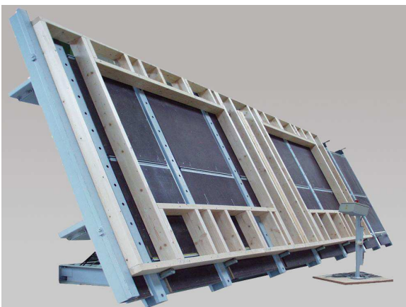
Bild 3: Zimmermeistertisch WTZ 110/10 LE
