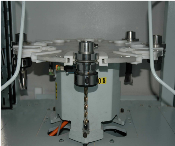
Bild 4: Sägezentrum WBS 140 mit Werkzeugwechsler
