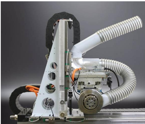
Neues Formfräsaggregat FK30 profiTrim
